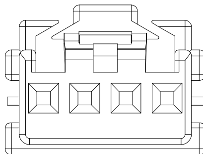
4Pin
