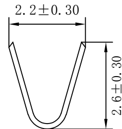
A-A SECTION
