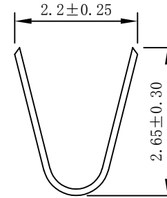
A-A SECTION
